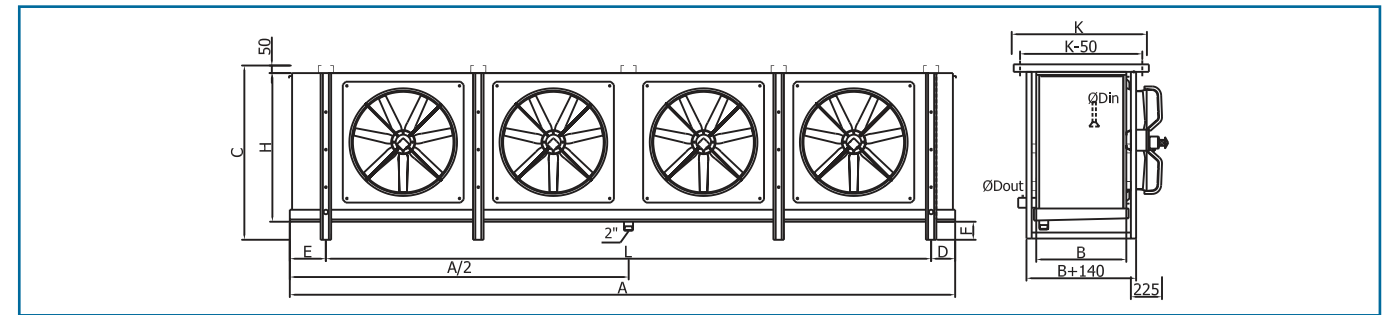
T SERİSİ fi OK DONDURUCU BOYUT TABLOSU T SERIES BLAST FREEZER DIMENSION TABLE • T SERIE SHOCKFROSTER MAßE
