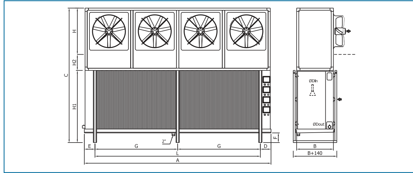
S ve H SERİSİ fi OK DONDURUCU BOYUT TABLOSU S and H SERIES BLAST FREEZER DIMENSION TABLE • S und H SERIE SHOCKFROSTER MAßE
