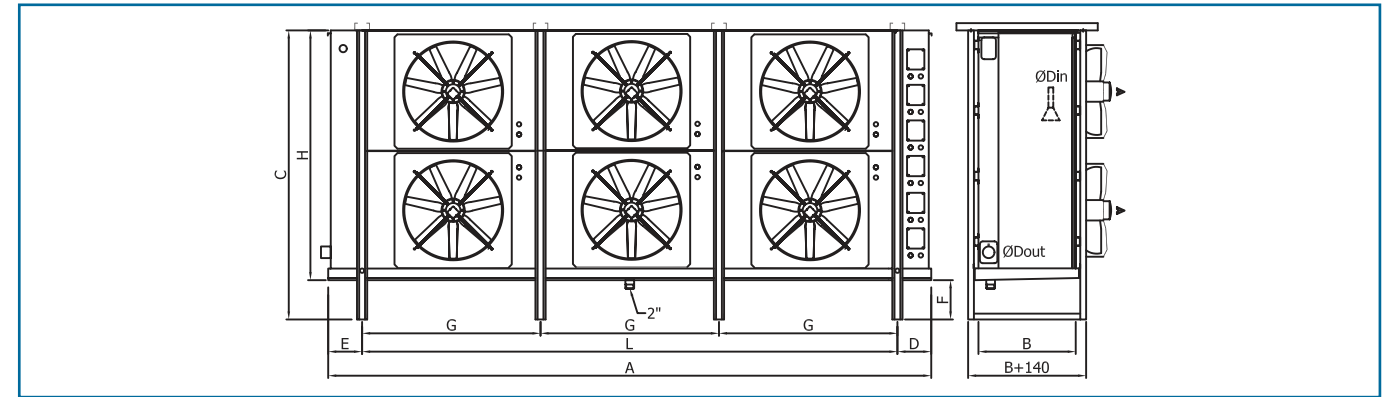
K SERİSİ fi OK DONDURUCU BOYUT TABLOSU K SERIES BLAST FREEZER DIMENSION TABLE • K SERIE SHOCKFROSTER MAßE
