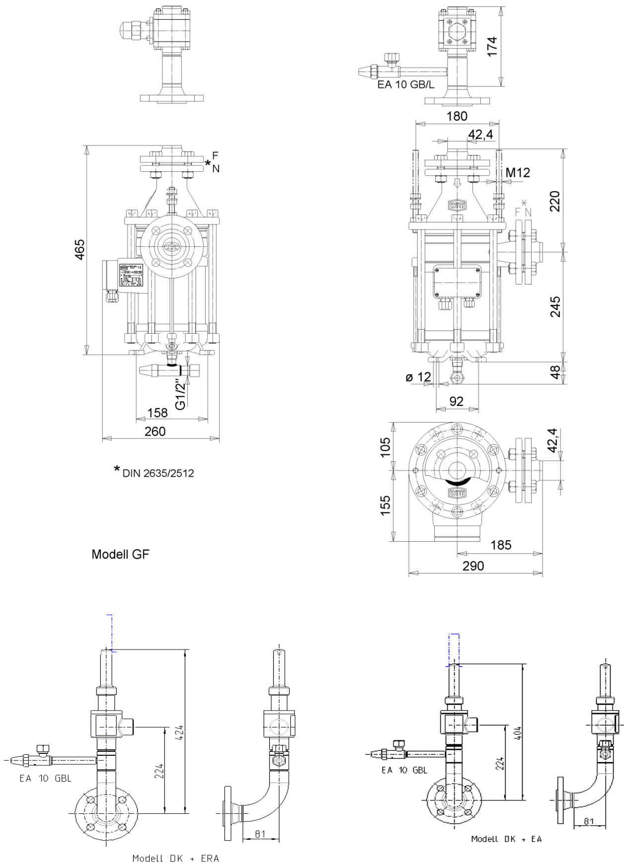
Fig. 1 HRP 3232
